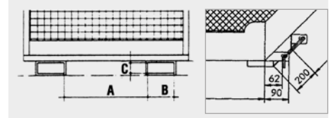
Einfahrtaschen-Innenmaße (mm)
