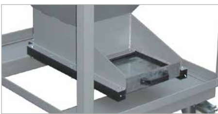
Schieberverschluss (SR-D, SG-D, SRE-D)
