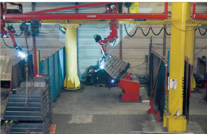
Schweißroboter-Anlagen
